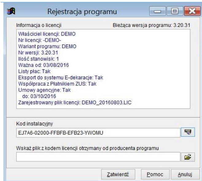
Rys.1. Rejestracja programu.
