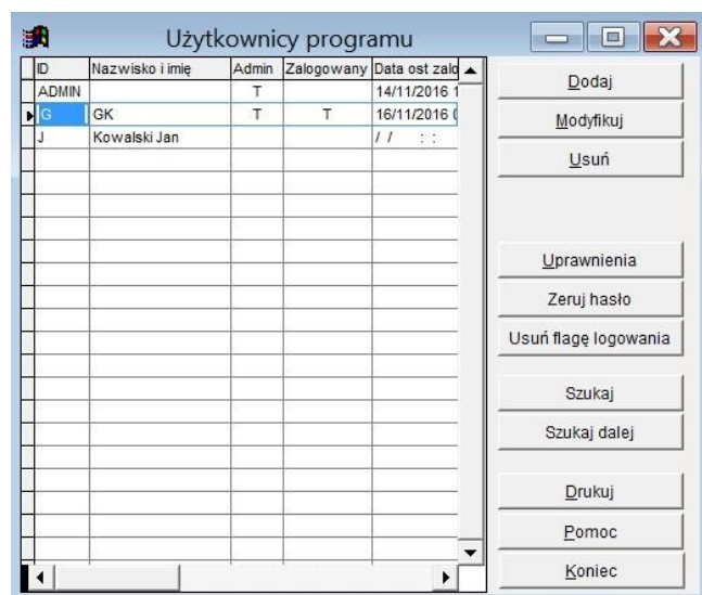
Rys.18. Lista użytkowników.
